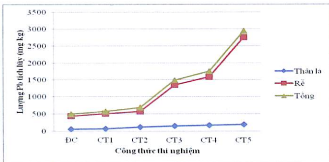
Hình 2. Ảnh hưởng của hàm lượng Pb trong đất đến lượng tích lũy Pb trong thân lá và rễ cây cỏ mần trầu.
